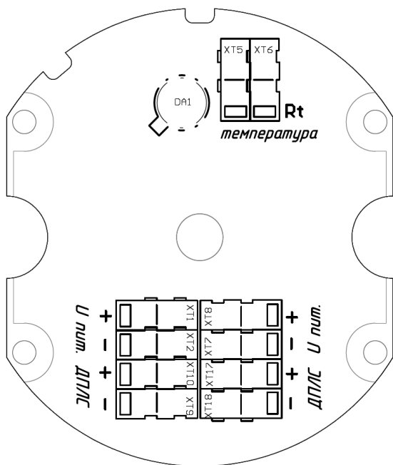
Рис.Б3. Внешний вид платы управления и схема подключения адресного извещателя ИП101 «Азимут» МК-АМ
