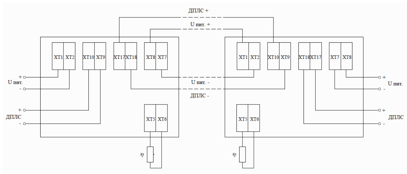
Рис.Б3. Внешний вид платы управления и схема подключения адресного извещателя ИП101 «Азимут» МК-АМ
