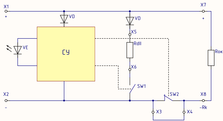
Параллельное включение
