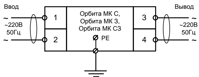
Схема подключения оповещателей Орбита МК С 220, Орбита МК 3 220, Орбита МК С3 220.
