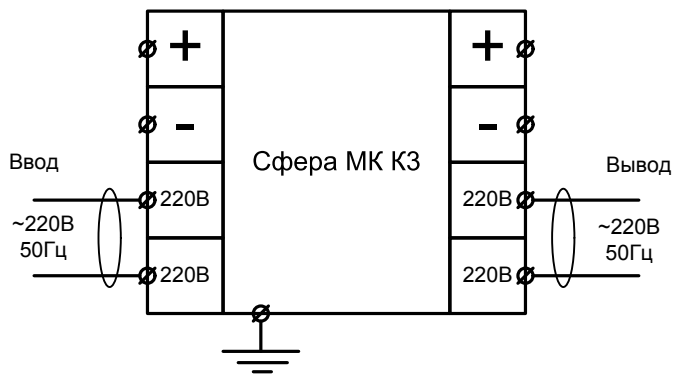
Схема подключения оповещателей Сфера МК Компл.3; питание переменным током
