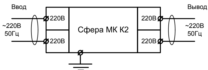
Схема подключения оповещателей Сфера МК Компл.2
