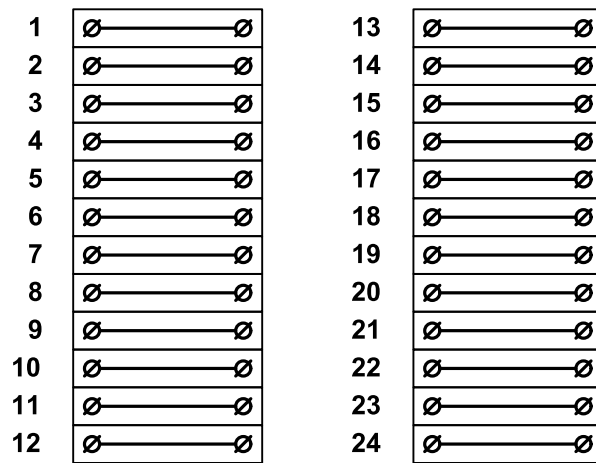
Монтажная коробка КВМК-тип Б. Схема монтажных клемм.
