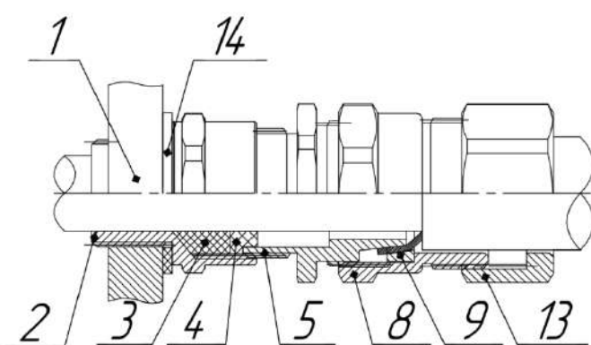
Прокладка бронированного кабеля
