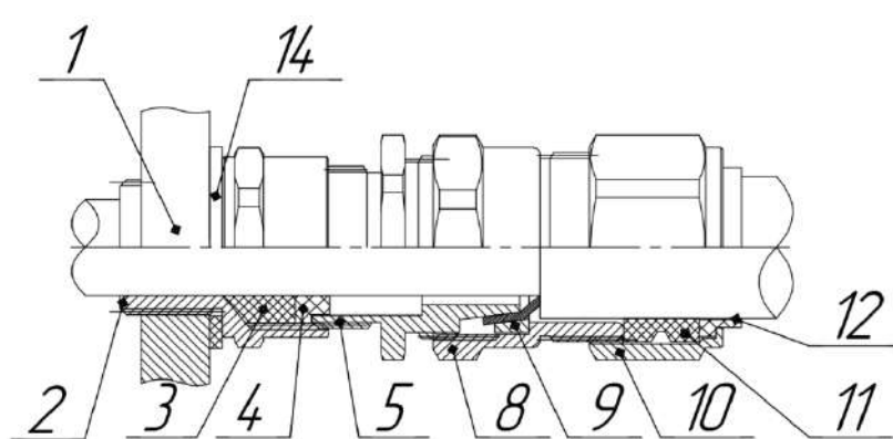
Прокладка бронированного кабеля с двойным уплотнением
