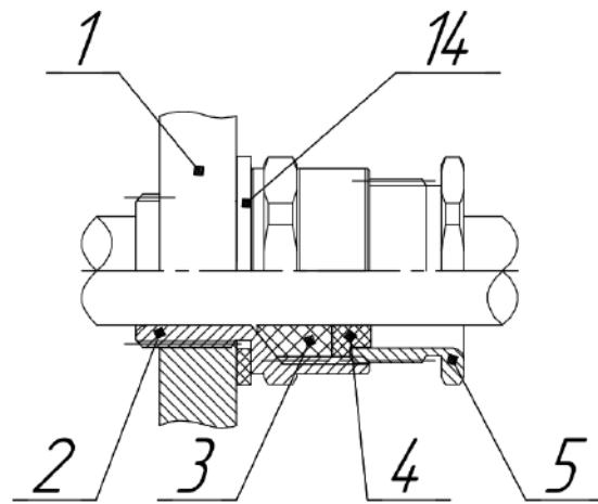
а) открытая прокладка кабеля
