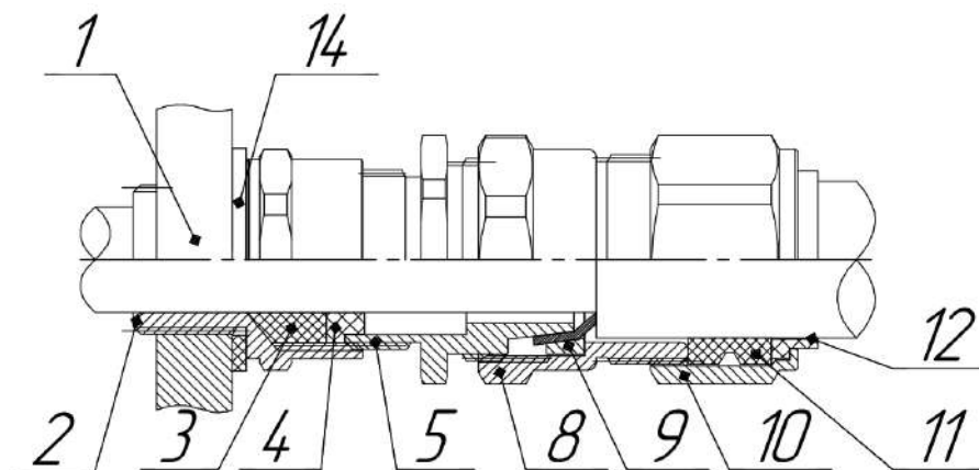
д) прокладка бронированного кабеля с двойным уплотнением
