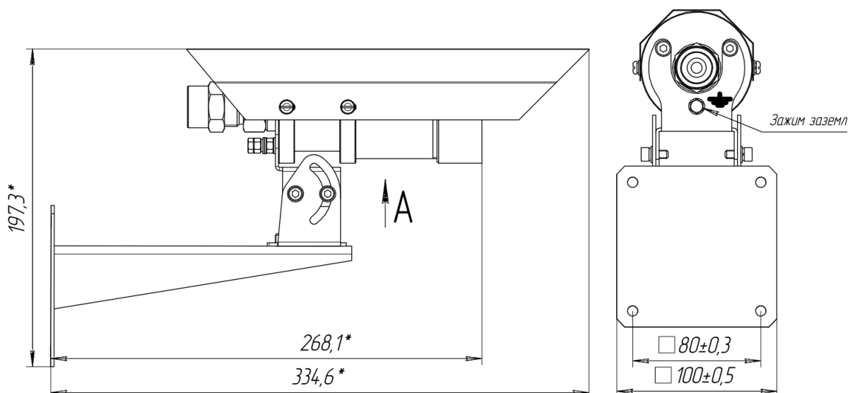
Рис.1 Общий вид компонентов извещателя ИП212 Трион-Л2 МК
