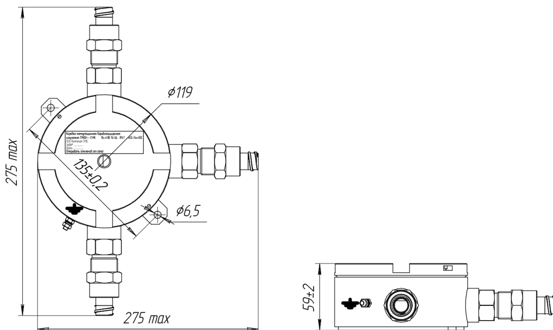
Рис.2 Габаритные и установочные размеры блока излучателя (приемника) извещателя ИП212 Трион-Л2 МК.
