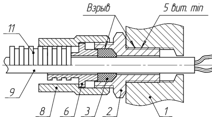
г) Ввод кабеля в металлопункте
