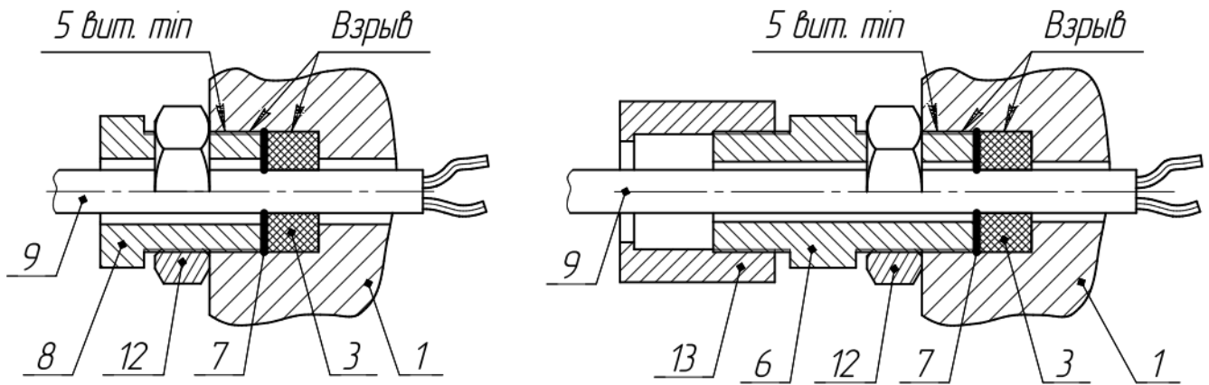
а) Открытая прокладка кабеля
