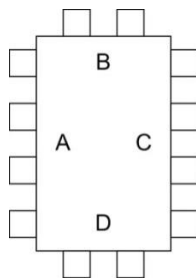
Рис. 1. Схема расположения вводов или отверстий в корпусе КВМК Ехе-II-XXX... X, СМД МК Ехе-II-XXX... X.
