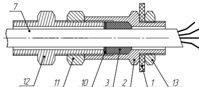
г) Кабель в трубе
