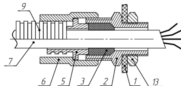
б) Кабель в металлорукаве
