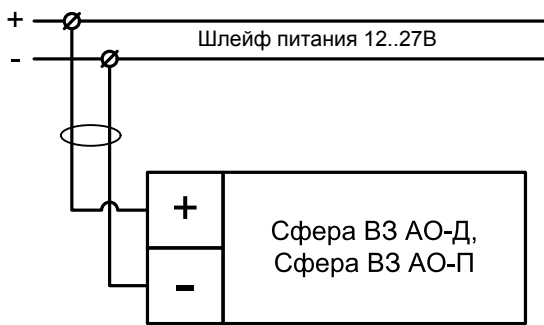
Схема подключения аварийных светильников Сфера В3 АО-Д, Сфера В3 АО-П
