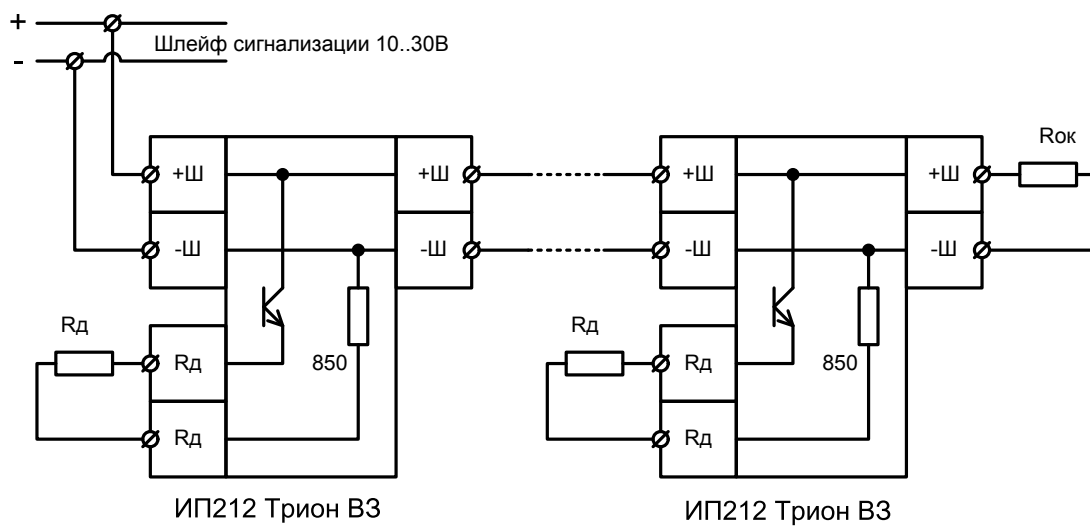
Схема подключения извещателя дымового ИП212 Трион В3.
