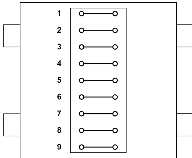
Монтажная коробка KBB3-тип A 1ExeIBT5Gb. Схема соединений. Клеммные зажимы WAGO 261: 24А; 500В; 2,5мм 2 .
