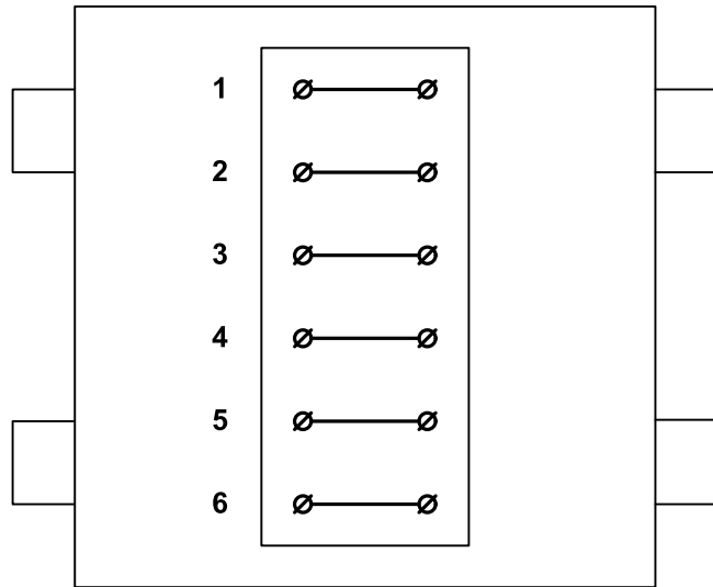
Монтажная коробка KBB3-тип A 0ExiaIBT5Ga. Схема соединений. Винтовой клеммный блок: винты М3; сечение 2мм 2 .
